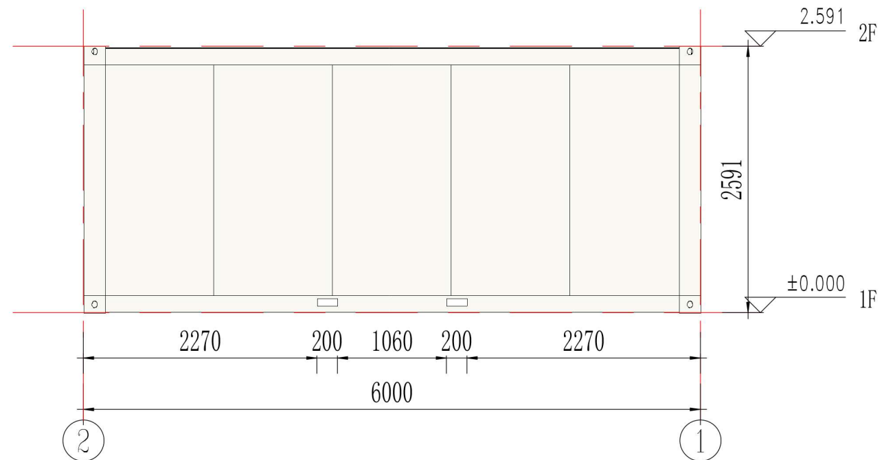
Élévation Nord
