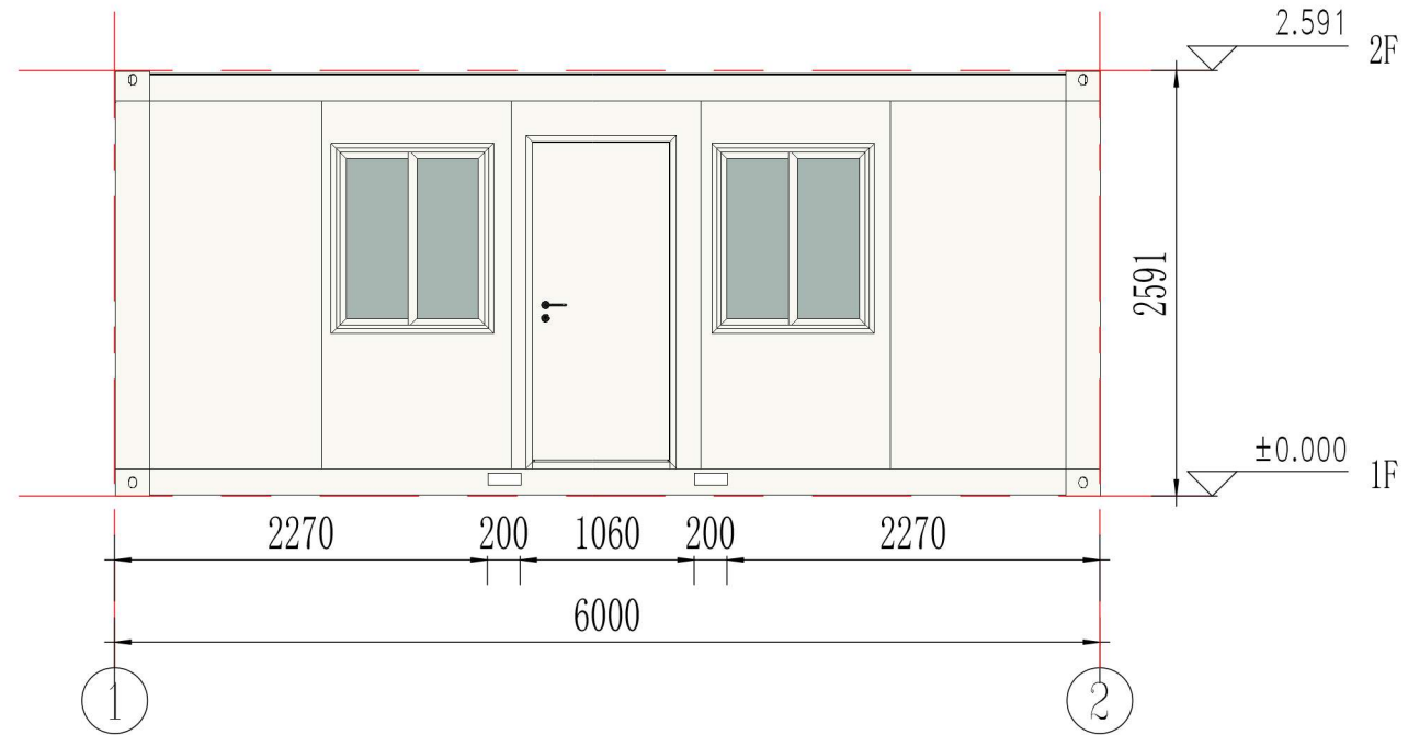
Élévation Sud
